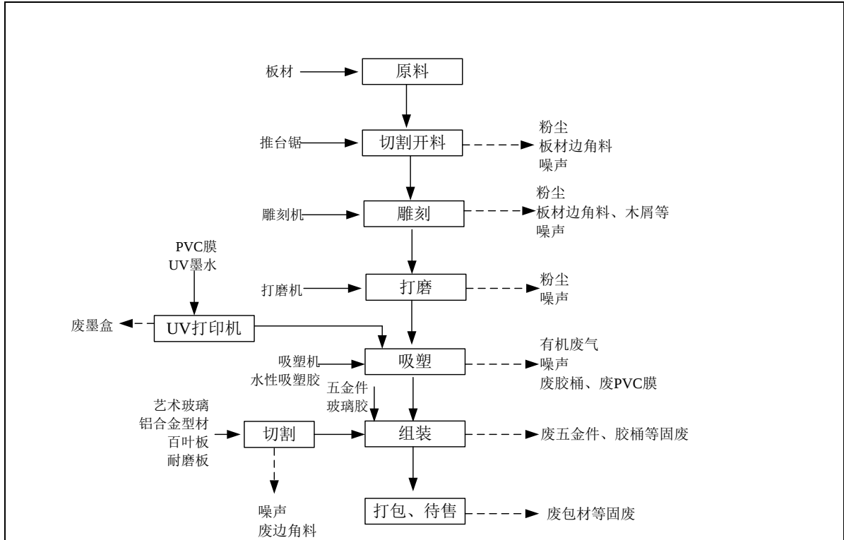
图 5-8 衣柜门生产工艺流程及产污环节图
