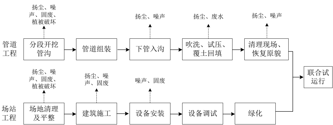
图 5-1 施工期施工工艺流程及产污位置图
