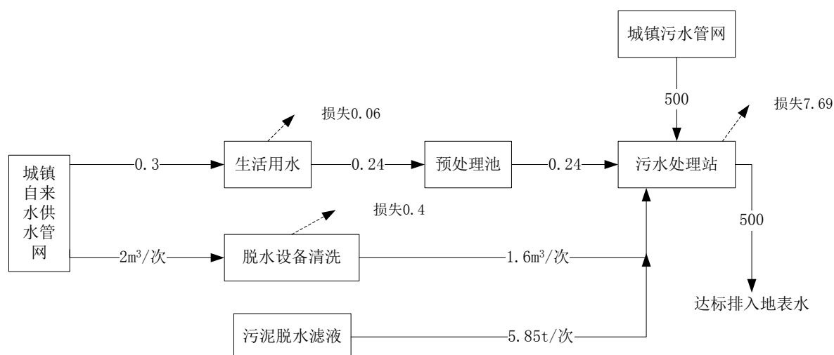
图 1-1 项目水平衡图单位：m 3 /d
