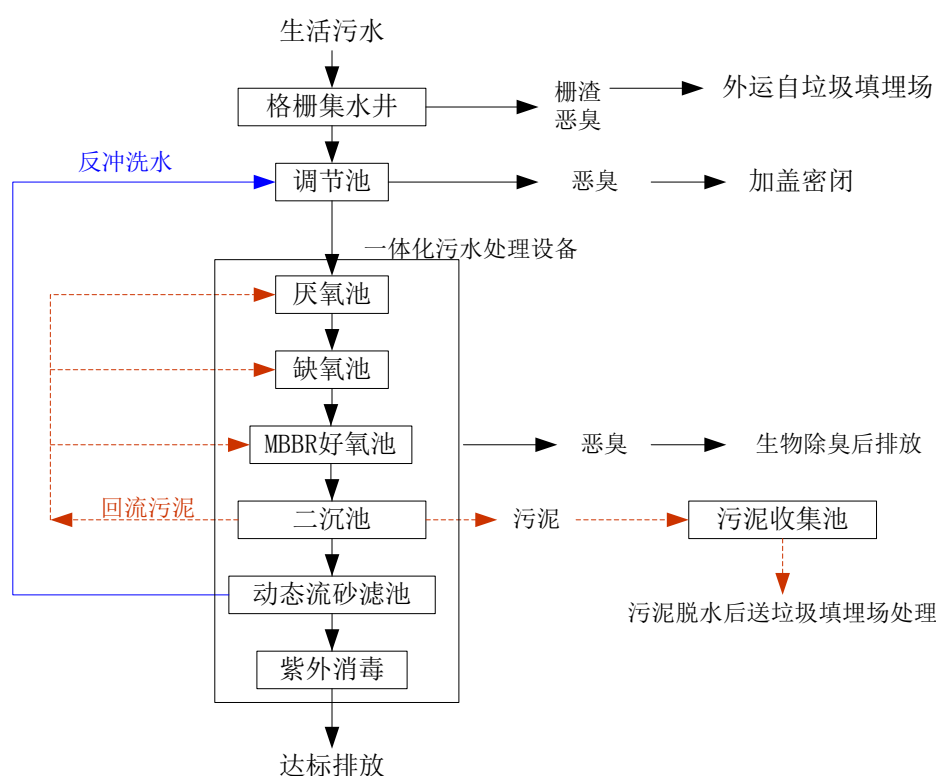
图 5-2 项目污水处理流程及产污节点图
