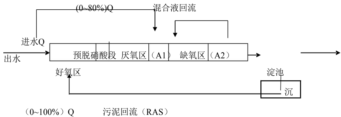
图3.2-3 改良A/A/O法工艺流程图
