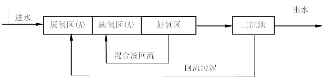
图3.2-1 A/A/O工艺流程图
