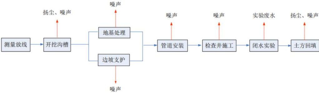
图3.2-6 管线工程施工期工艺流程图
