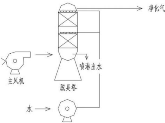
图8.1-1生物滤池脱臭工艺流程图
